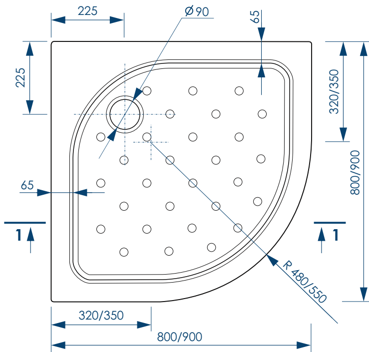
Вид сверху
