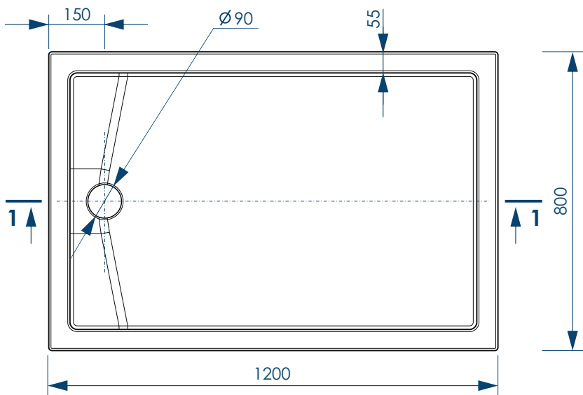
Вид сверху
