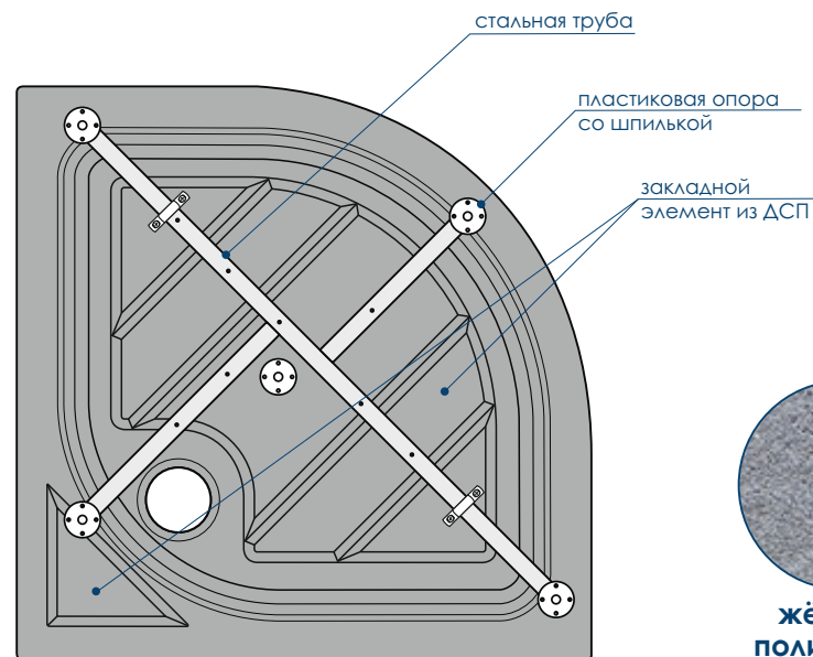
Вид снизу
