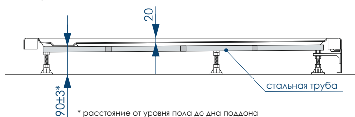
Разрез 1-1
