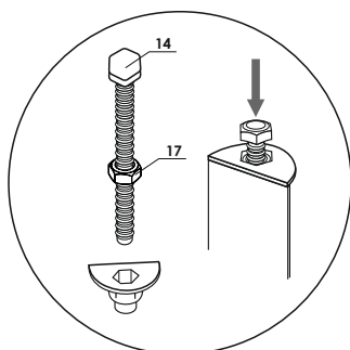
Верхняя ножка
