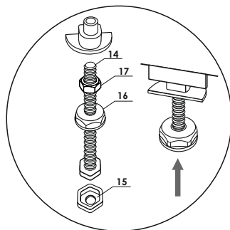
Нижняя ножка
